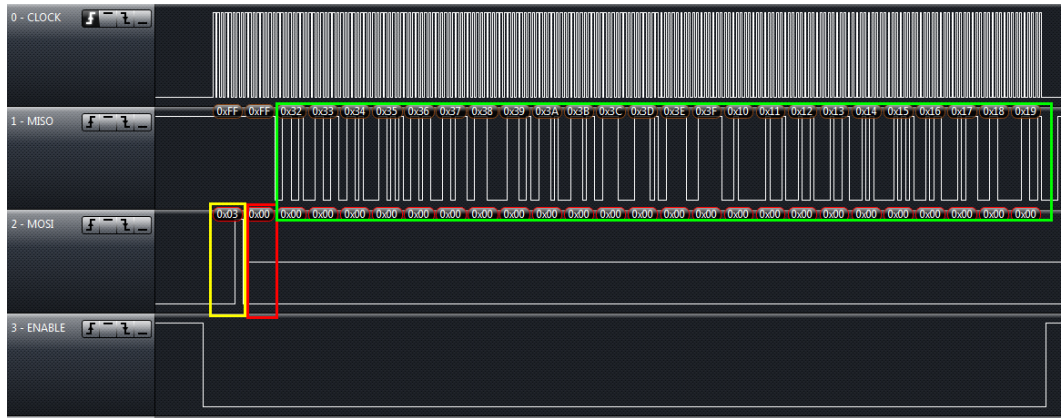
图 4-6. 波形图 2
