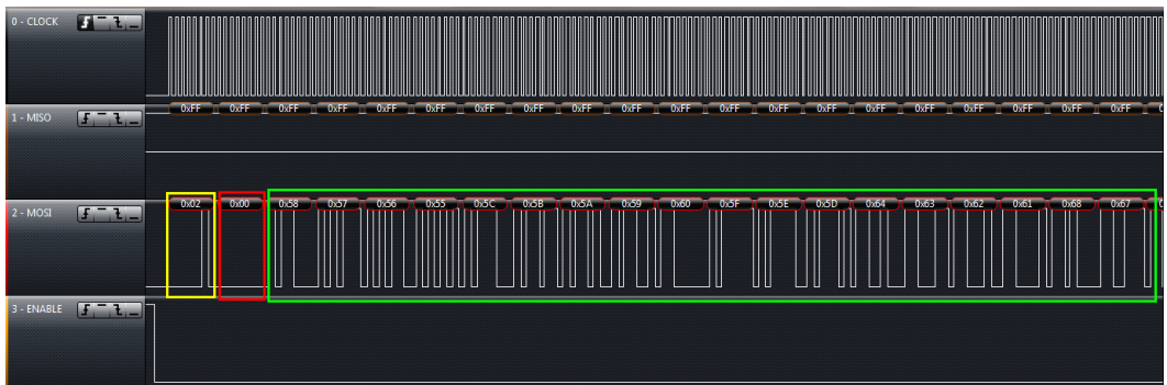
图 4-5. 波形图 1
