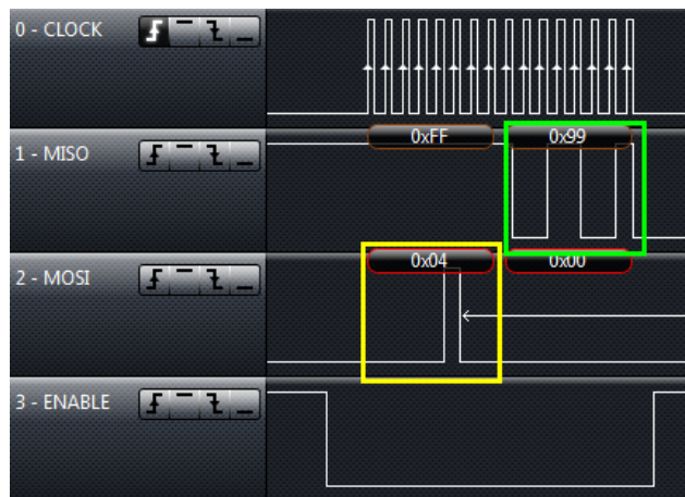
图 4-7 波形图 3
