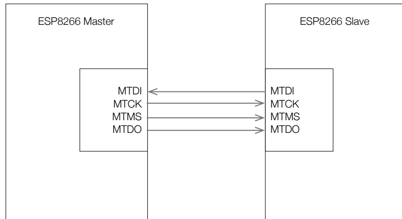
图 4-3. 测试 Demo 硬件连接图
