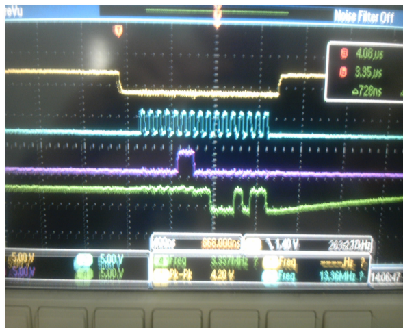
图 4-2. spi_byte_read_espslave 读取 ESP8266 从机波形
